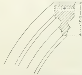
Fig. 11. Żebro kaplicy Marjačkiej.
